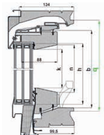
Attālums starp kārbas frēzējumiem - vertikāli mm (q)
